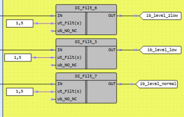
Датчики уровня для осушения резервуара
