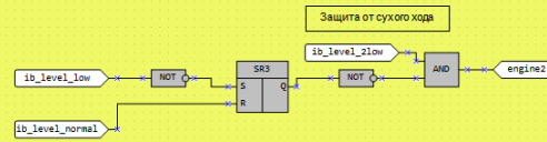
Алгоритм осушения бака с защитой от сухого хода насоса
